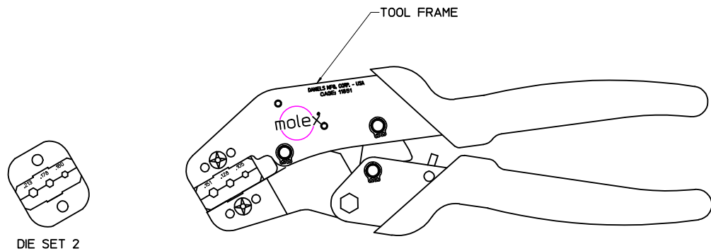
DIE SET 2
