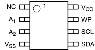
SOIC (W, X), TSSOP (Y), UDFN (HU5)
